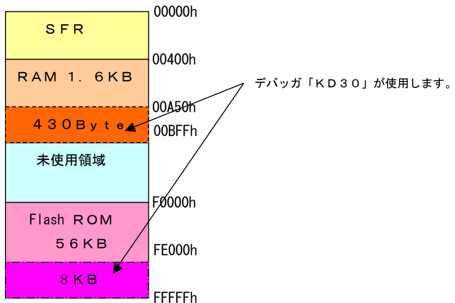
図7 OAKS16-MINIのメモリマップ
