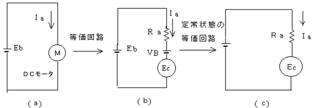
図18 DCモータの等価回路
