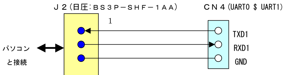
図9 RS-232Cの接続
