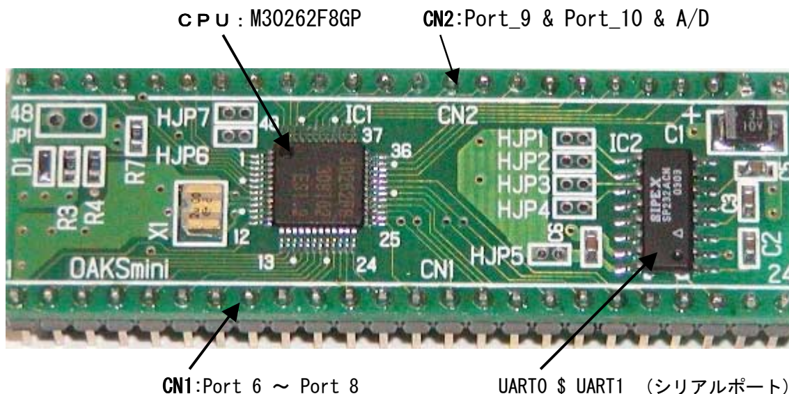
図8 OAKS16-MINI CPUボード
