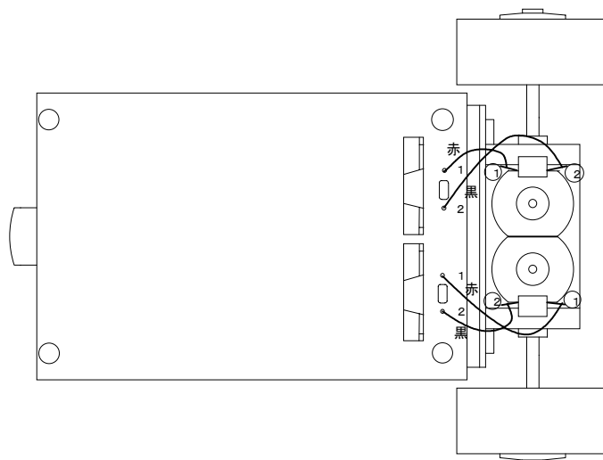
モータ 配線
