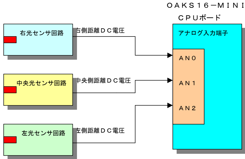
図 2 0 光距離センサ回路と A/D 変換器の接続
