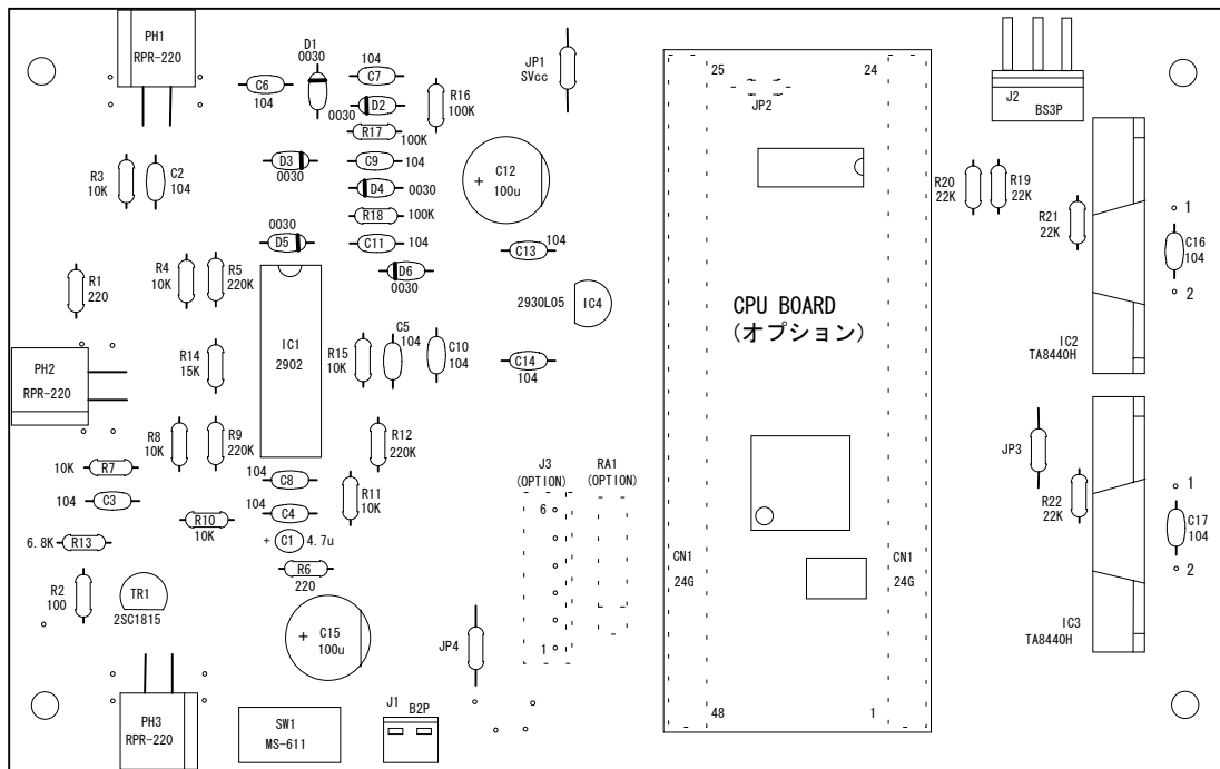
OAKS16-Mini (M30262F8GP) 用 SENSOR LABO 基板実装図
