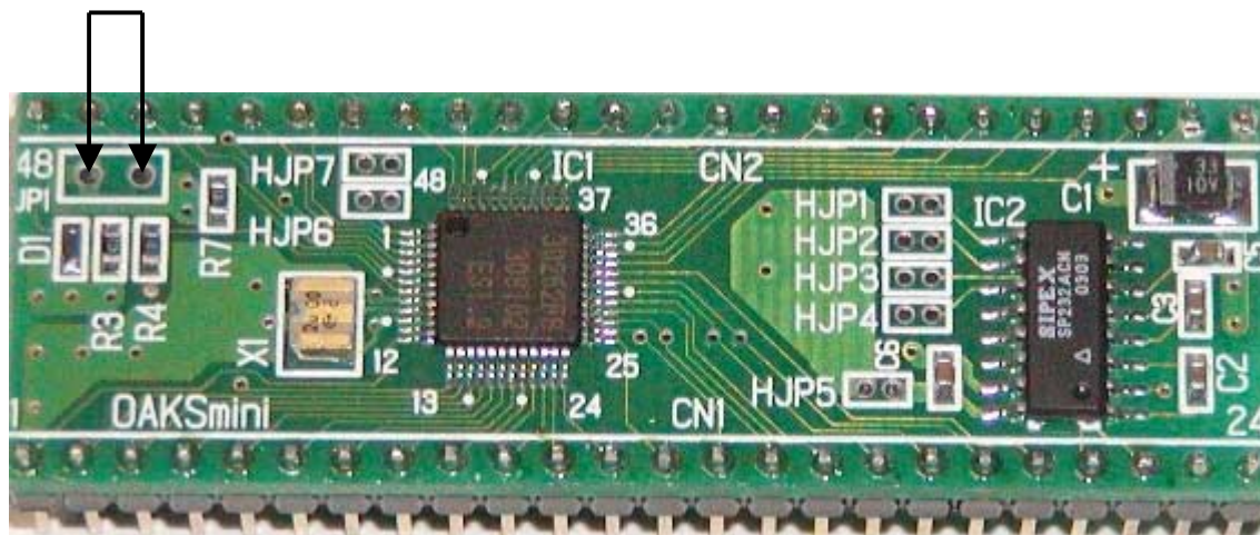
図31 CPUボード「OAKS16-MINI」のJP1端子
