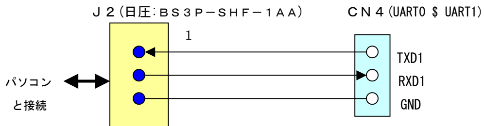
図9 RS-232Cの接続
