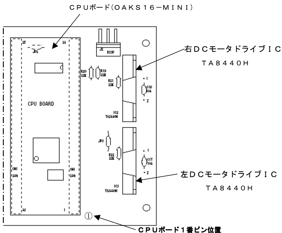
図1 モータドライブ部の構成図
